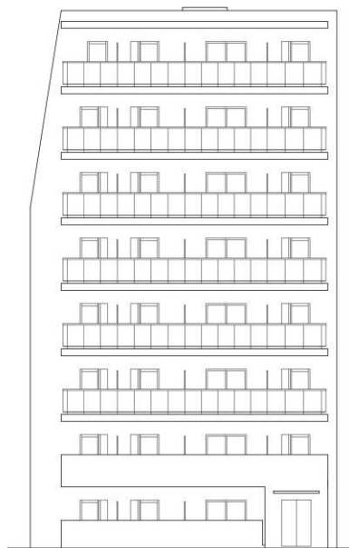
南側立面図
