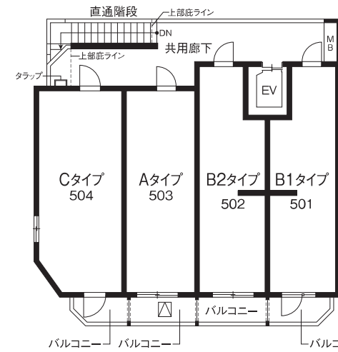
5F 平面図
