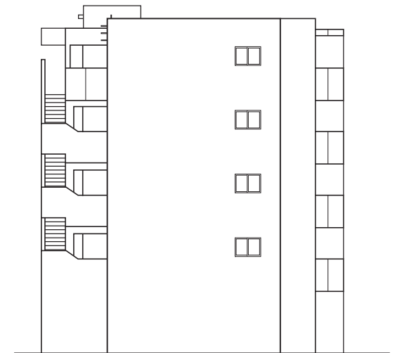
東立面図
