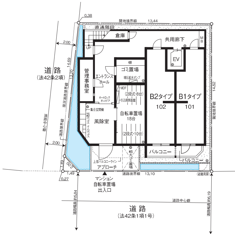
1F 平面図
